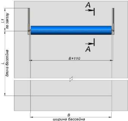
Скиммерный бассейн Вид сверху
